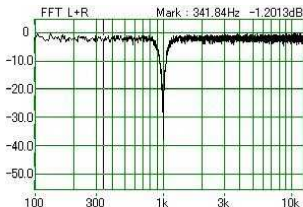
図12 高域半波長遅延
