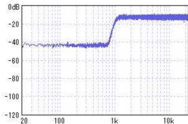
図 13 ゲイン調整無し
